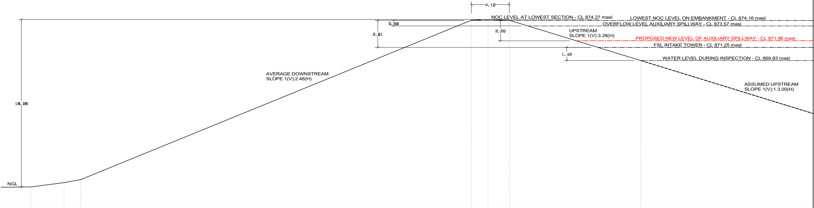
EMBANKMENT LONGITUDINAL SECTION (A-A) - SCALE (V) 1:100 (H) 1:1000 (A3)
